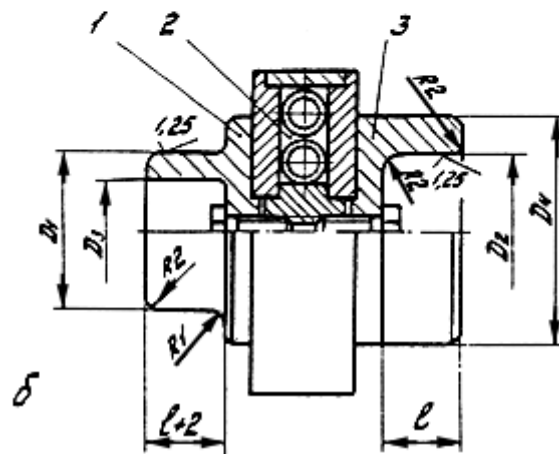
Рис. 10. Схема нагревательного инструмента для раструбно-стыковой сварки: а - газопламенного нагрева; б - с электрическим нагревом и сменными деталями; 1 - дорн; 2 - электрический нагреватель; 3 - гильза
