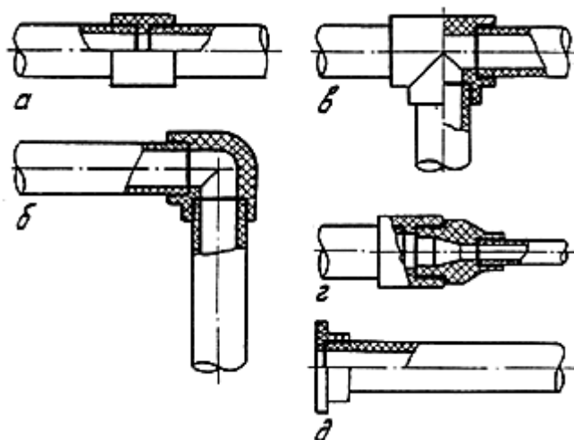
Рис. 6. Сварные раструбно-стыковые соединения труб и соединительных деталей из ПВХД:
