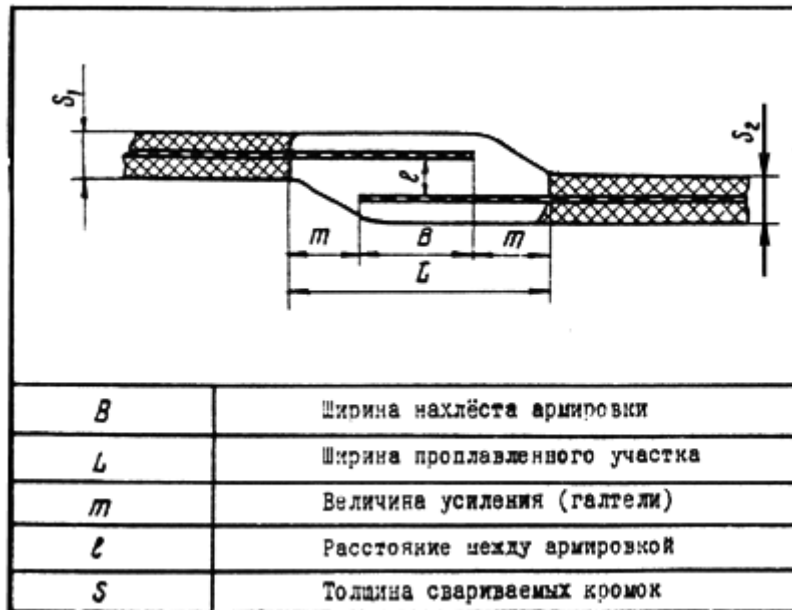
Конструктивные элементы сварного шва
