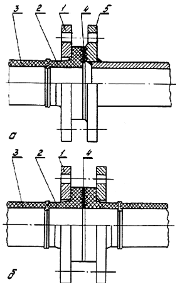
Рис.11. Фланцевые соединения:
