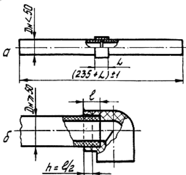
Рис. 2. Образцы для испытаний сварных раструбных соединений:
