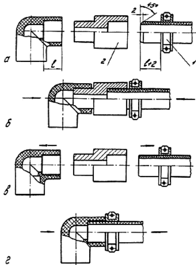
Рис. 9. Последовательность процесса контактной сварки впаструб труб и соединительных деталей из ПВД:
